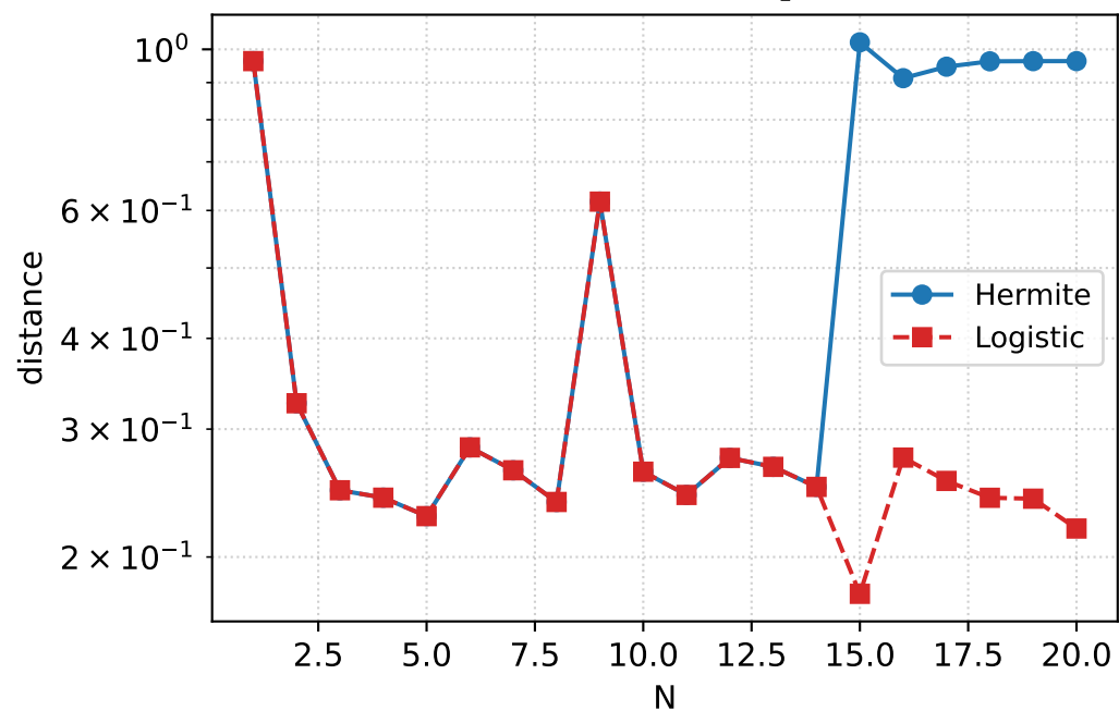
(d) L2 distance d_2
